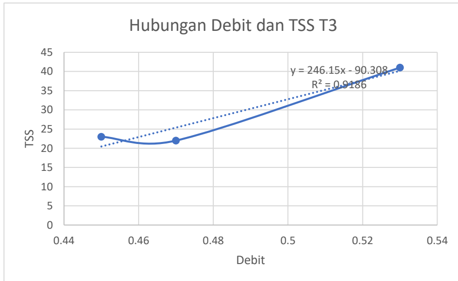
Gambar 6. Hubungan antar debit dan TSS T3
