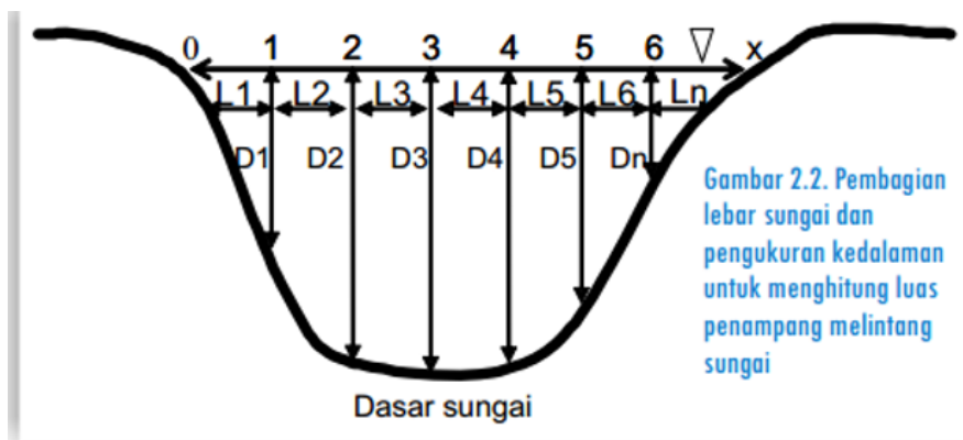
Gambar 2. Gambaran penampang sungai
