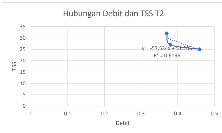
Gambar 5. Hubungan antara debit dan TSS T2
