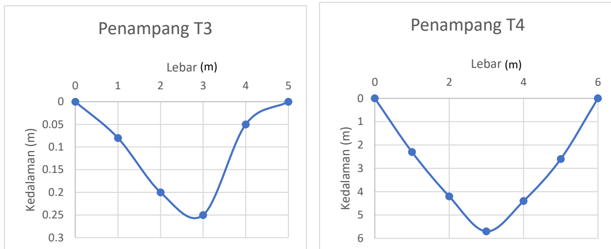
Gambar 3. Profil penampang sungai
