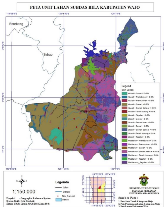
Gambar 1. Peta unit lahan Sub-DAS Bila
