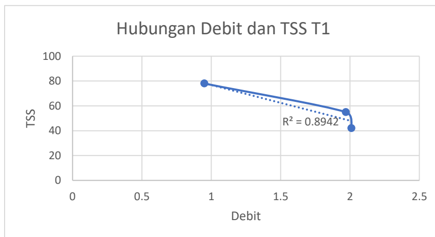
Gambar 4. Hubungan antara debit dan TSS T1
