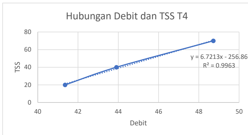
Gambar 7. Hubungan antara debit air dan TSS T4
